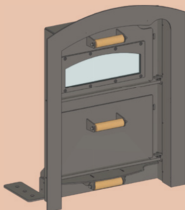
Backofentür WBT42D
