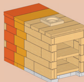
REMUS Duo 60120
