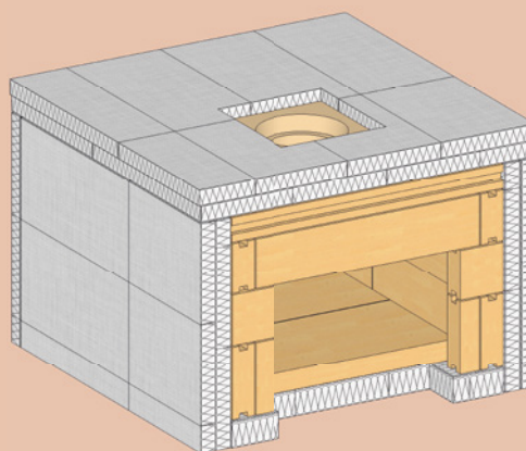
8 cm Wand- und Deckendämmung
