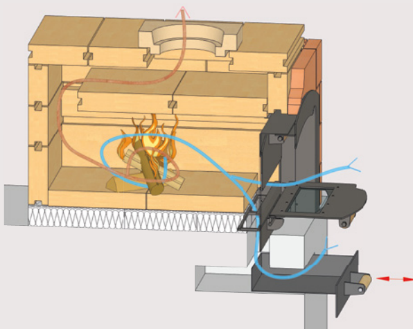
Verbrennungsluftführung
