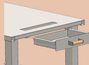
Metallsockel mit individuell angebrachten Führungsschienen
