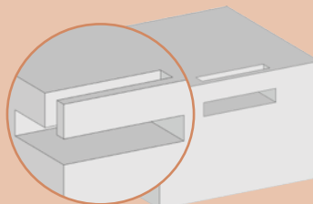
Aschefach im gemauerten Sockel
