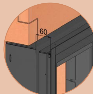
Blendrahmen 60 mm tief
