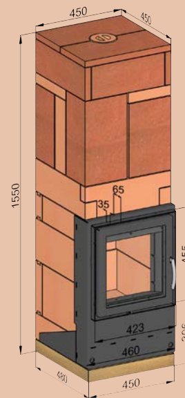
Maße Version OI/60
