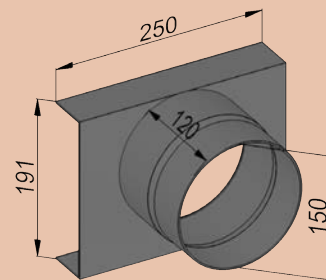
Zuluftstutzen
