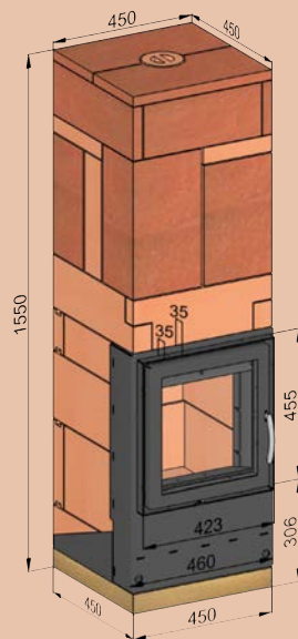
Maße Version OI/30
