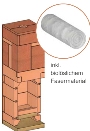
Innenausbau Speicherofen HÖLZLI OI/30 Speicherofen HÖLZLI OI/60
