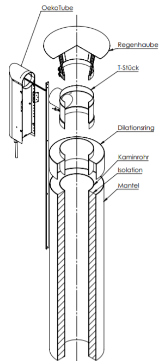
OekoTube-Outside , Edelstahlkamin
