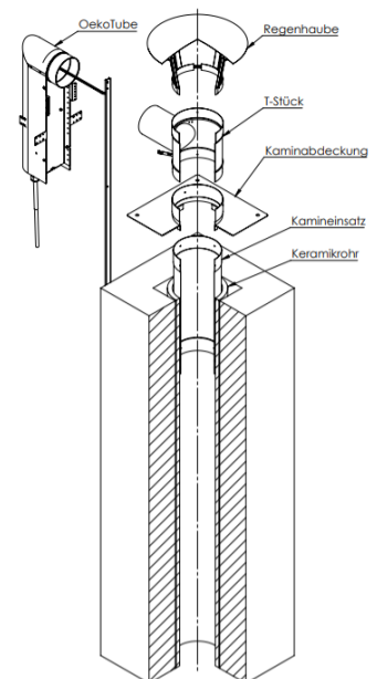
OekoTube-Outside, Mauerwerkschornstein, keramischer Schornstein
